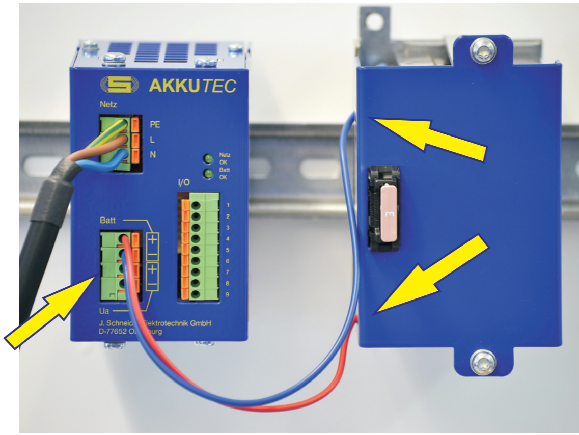
Anschluss des Akkus an den Batterieanschluss des AKKUTECH
