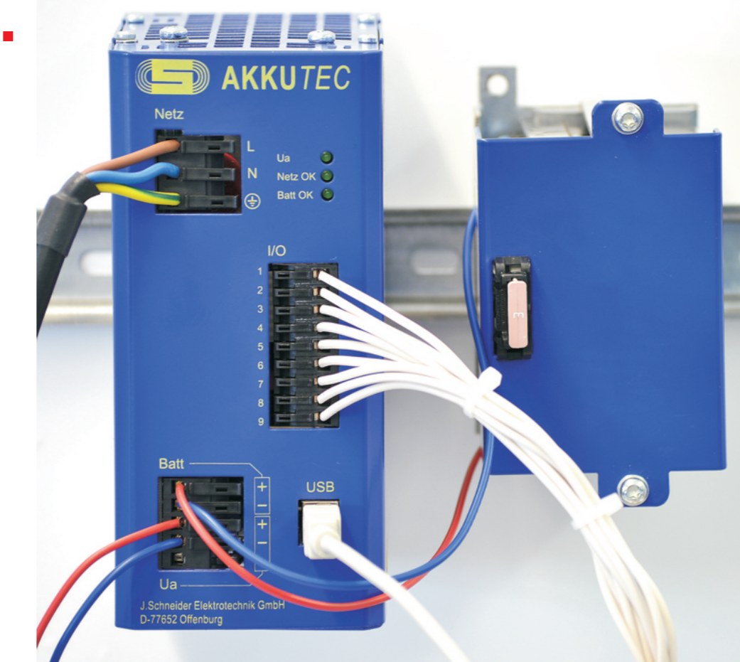
Anschluss der USB-Verbindung zum PC
