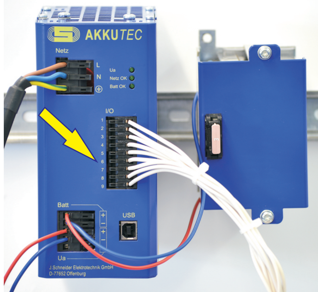
Verdrahtung der Ein-/Ausgänge (Temp. Sensor, Shutdown, Netz ok, Batt ok)
