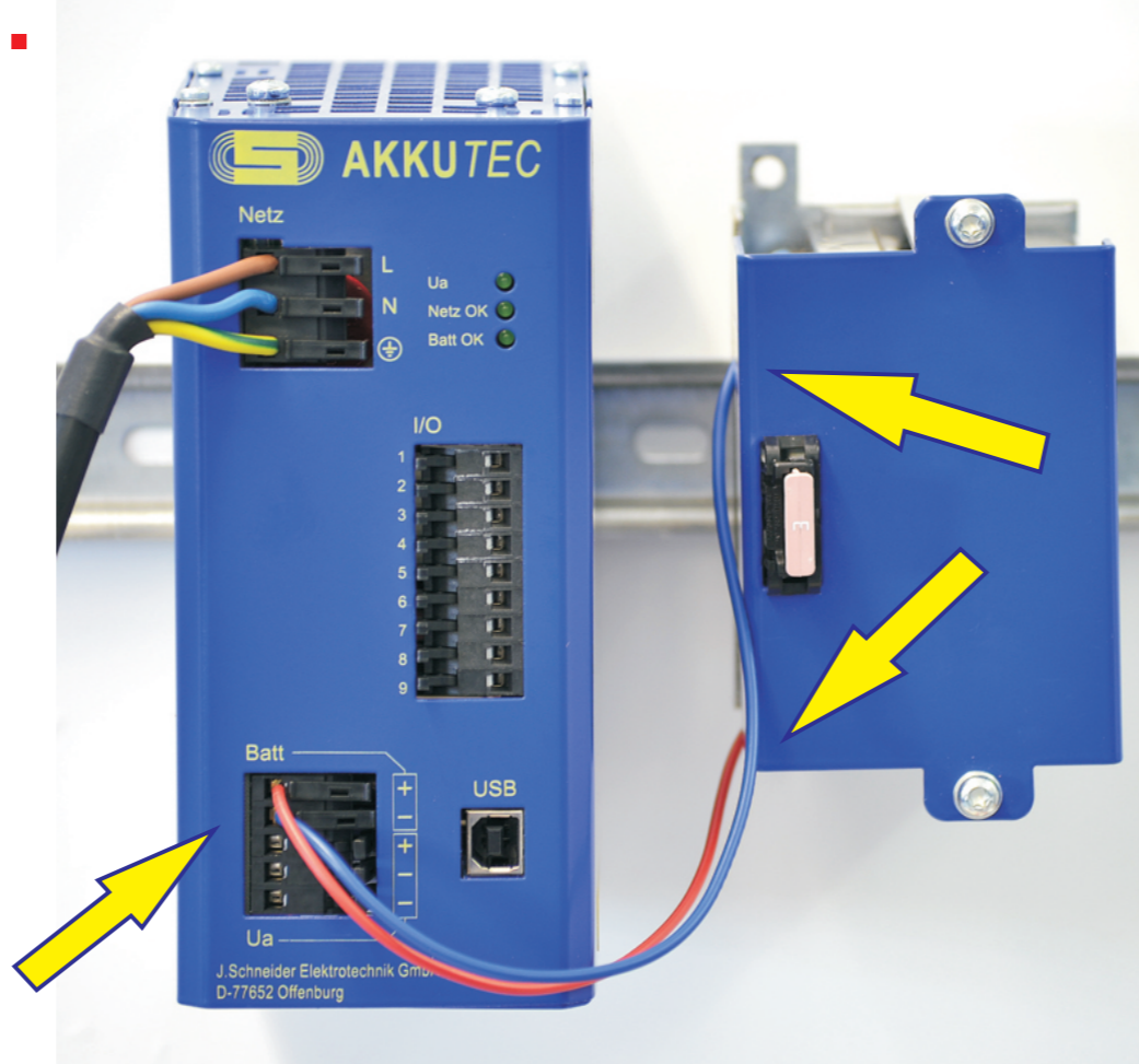
Anschluss des Akkus an den Batterieanschluss des AKKUTEK
